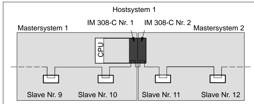
Bild 6-4 Multi-Master-Betrieb
