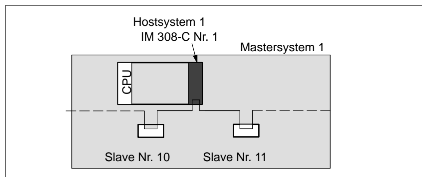
Bild 6-3 Mono-Master-Betrieb
