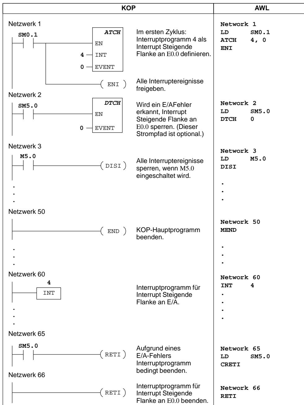
Bild 10-57 Beispiel für Interrupt-Operationen in KOP und AWL
