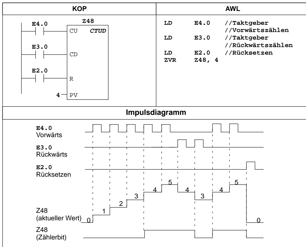
Bild 10-7 Beispiel für Zähloperationen in KOP und AWL
