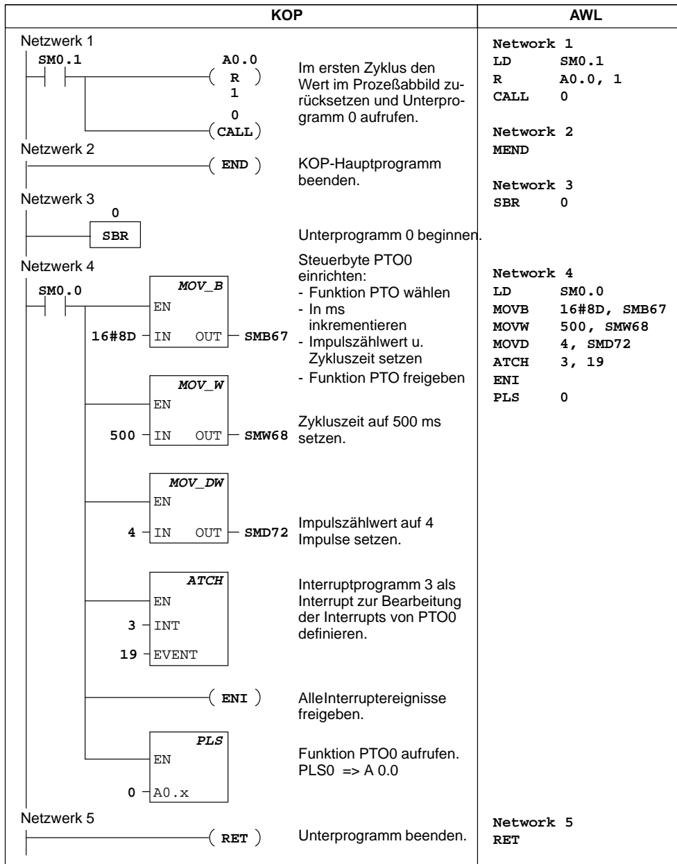
Bild 10-18 Beispiel für eine Impulsfolge
