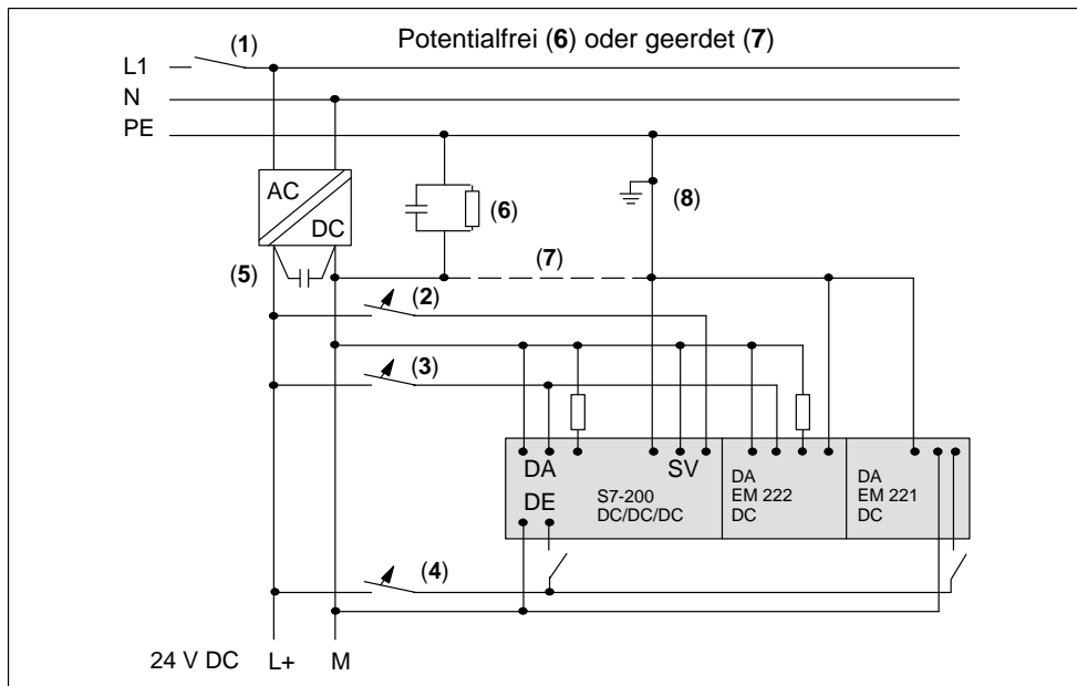
Bild 2-13 Isolierter DC-Aufbau
