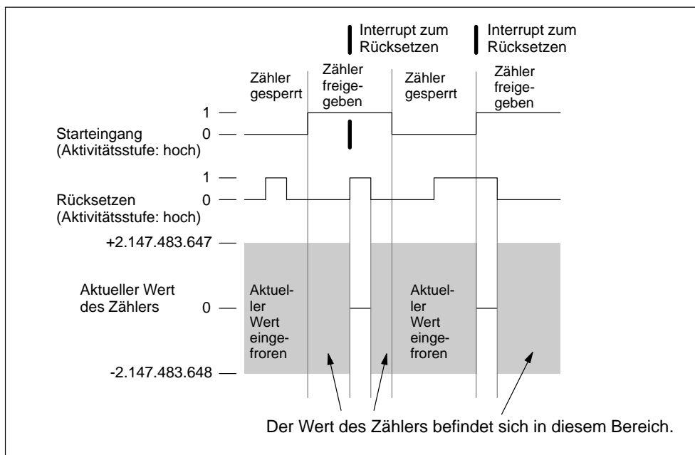
Bild 10-9 Beispiel für den Betrieb eines Zählers mit Rücksetz- und Starteingang
