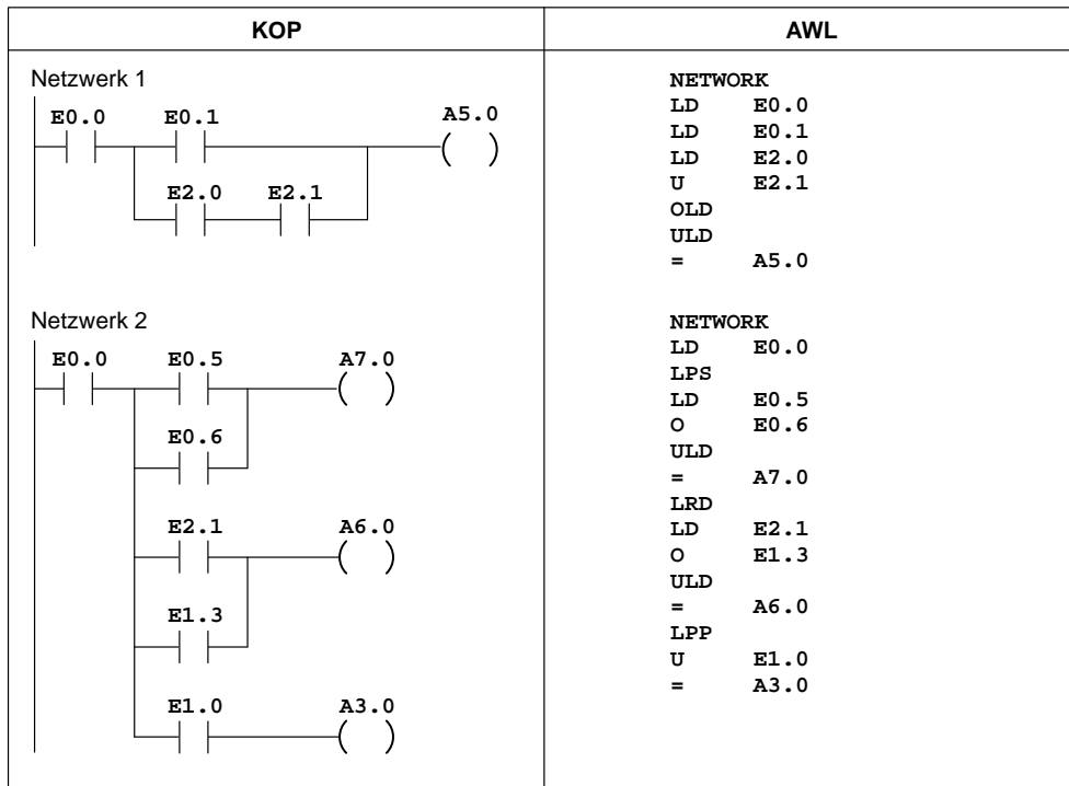
Bild 10-48 Beispiel für Stackoperationen in KOP und AWL
