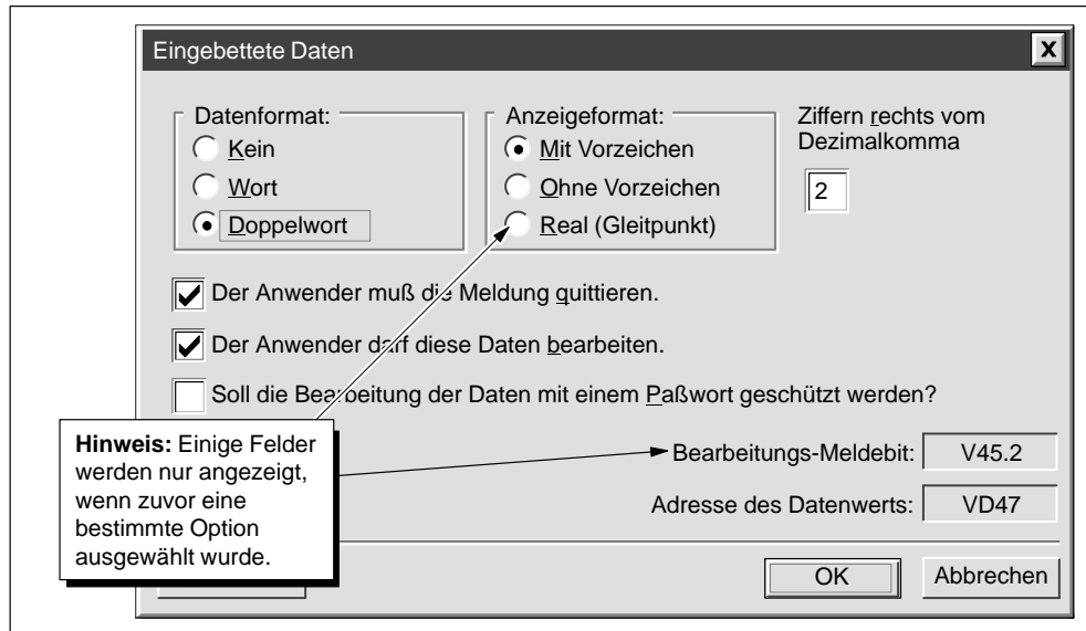
Bild 5-10 Dialogfeld "Eingebettete Daten" im TD 200-Assistenten
