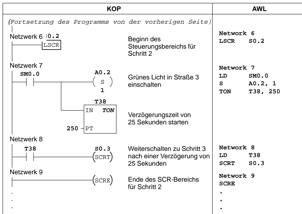
Bild 10-39 Beispiel für Ablaufsteuerungsrelais (SCR), Fortsetzung
